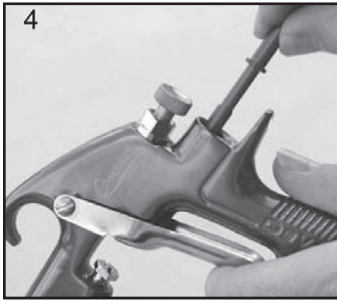
4. Remove Spindle (11).
